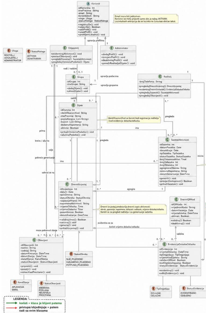
eVrtić sistem - finalni dijagram klasa
